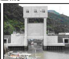
津波・高潮対策としての水門整備
